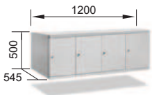
YK4/300
