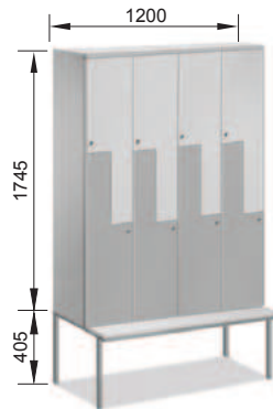
ZGKU4/300+SP
