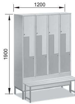
ZGK4/300+PP
