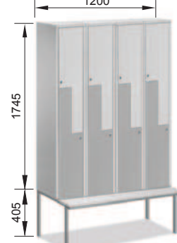
ZRKU4/300+SP
